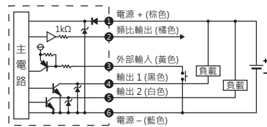
EFP02-□-010 NPN 輸出、類比電壓輸出與外部輸入型
