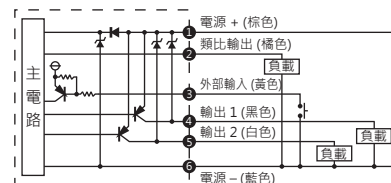
EFP02-□-031 PNP 輸出、類比電流輸出與外部輸入型
