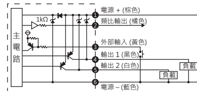
EFP02-□-030 PNP 輸出、類比電壓輸出與外部輸入型
