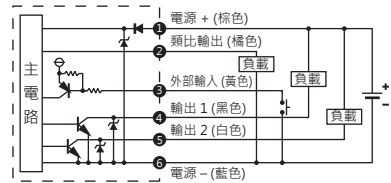
EFP02-□-011 NPN 輸出、類比電流輸出與外部輸入型
