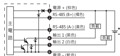
EFP02-□-02 NPN 輸出、RS-485 Modbus 通訊型
