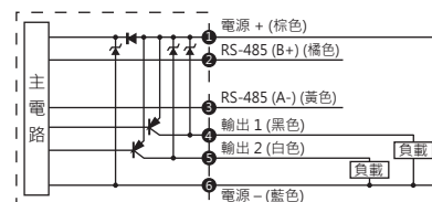
EFP02-□-04 PNP 輸出、RS-485 Modbus 通訊型
