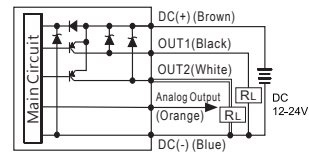
EP43 □ -04- □ 2 PNP+Copy Function
