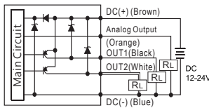
EP43 □ -031- □ 2 PNP+Analog Output (4~20mA)
