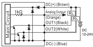
EP43 □ -010- □ 2 NPN+Analog Output (1~5V)
