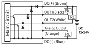
EP43 □ -011- □ 2 NPN+Analog Output (4~20mA)
