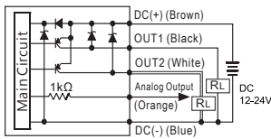
EP43 □ -030- □ 2 PNP+Analog Output (1~5V)
